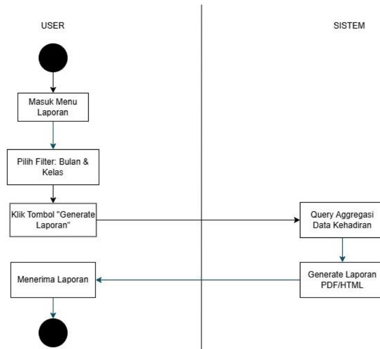
Gambar IV. 12 Activity Diagram Cetak Laporan Kehadiran
